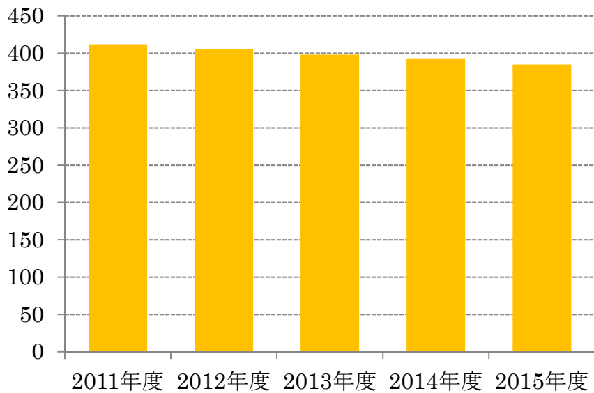
図 単位面積あたりの電力使用量[kWh/m 2 ・年]
