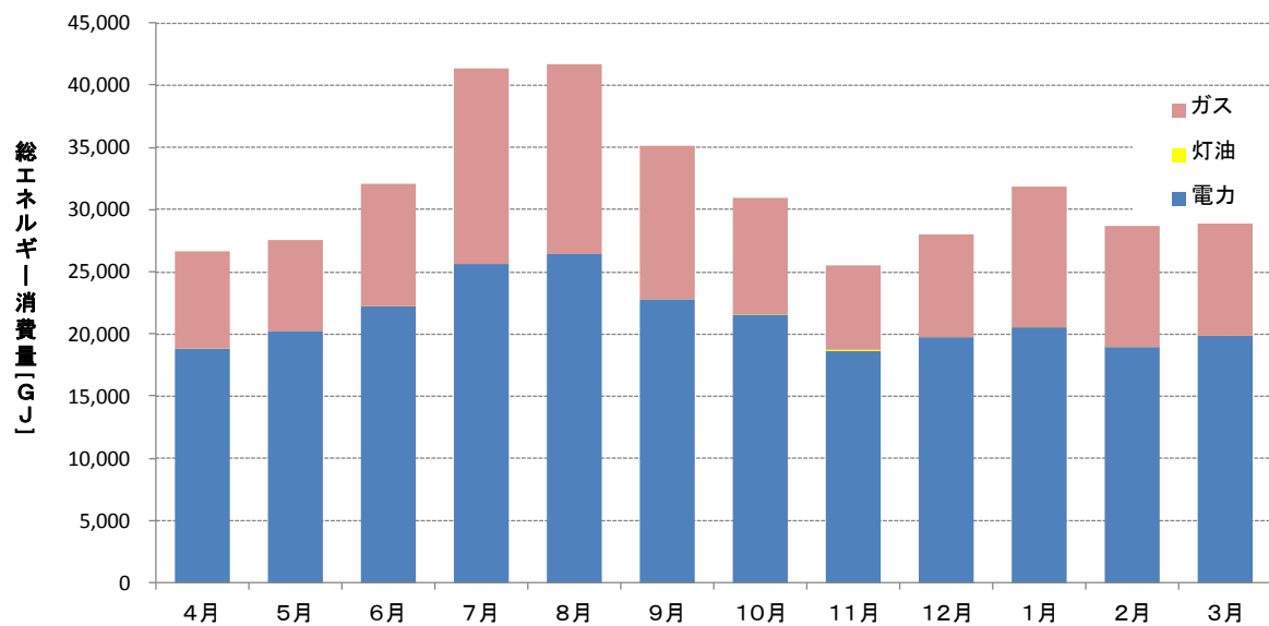
図 月別総エネルギー消費量 (2013 年度)
